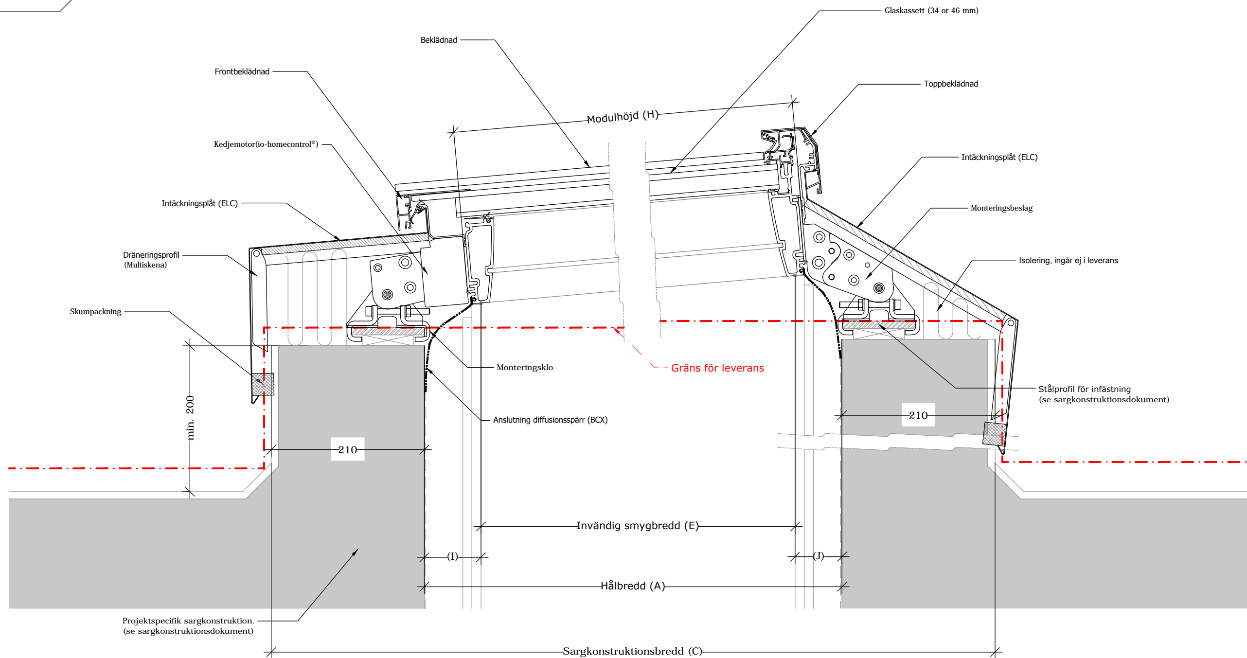
Sektionsvy - princip
